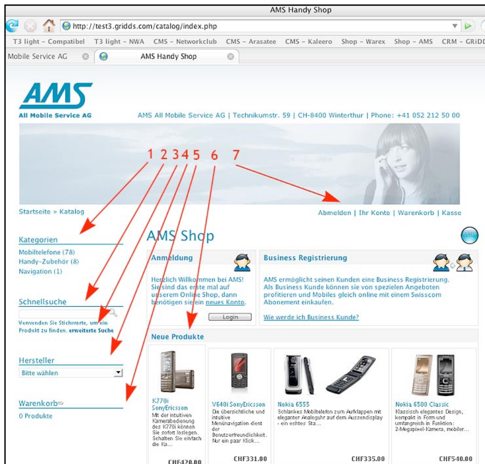
Abb.2 Startseite
