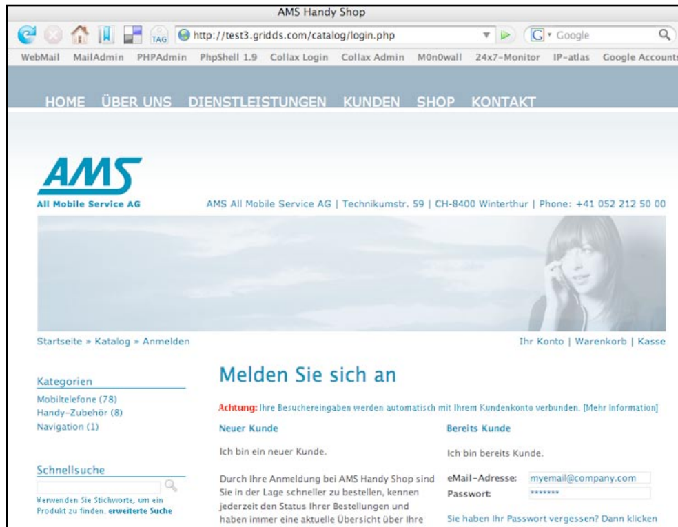
Abb.1 Login
